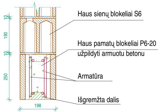
Pjūvis A-A
